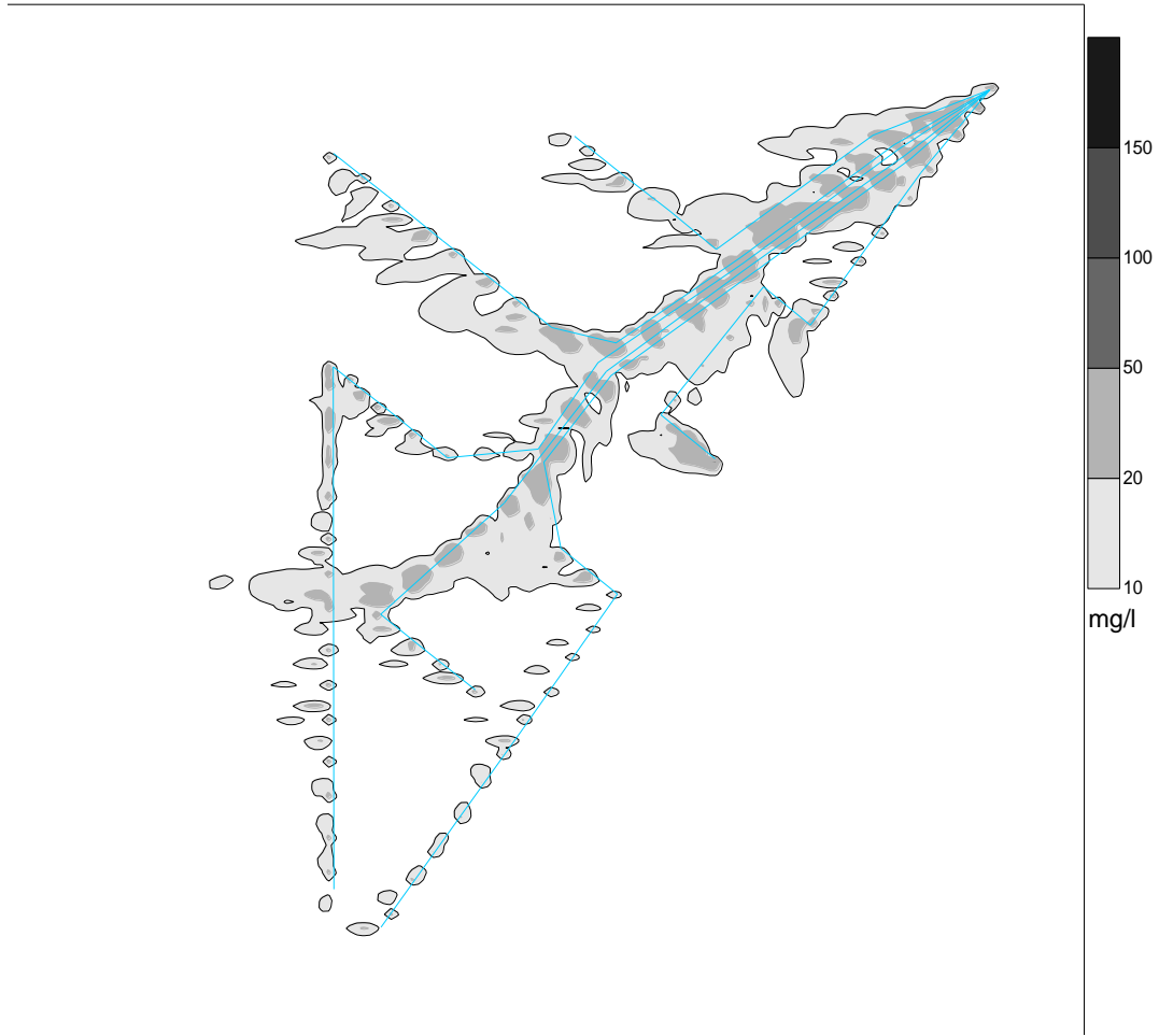
图 4.1.6-5 方案二 66KV 电缆铺缆次底层悬沙增量包络线（大于 10mg/L 面积 15.635km 2 ）
