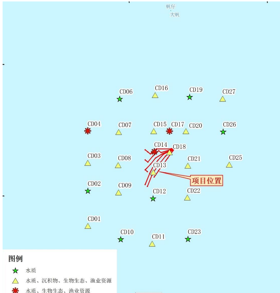
图 3.2.6-2 秋季调查站位布置图
