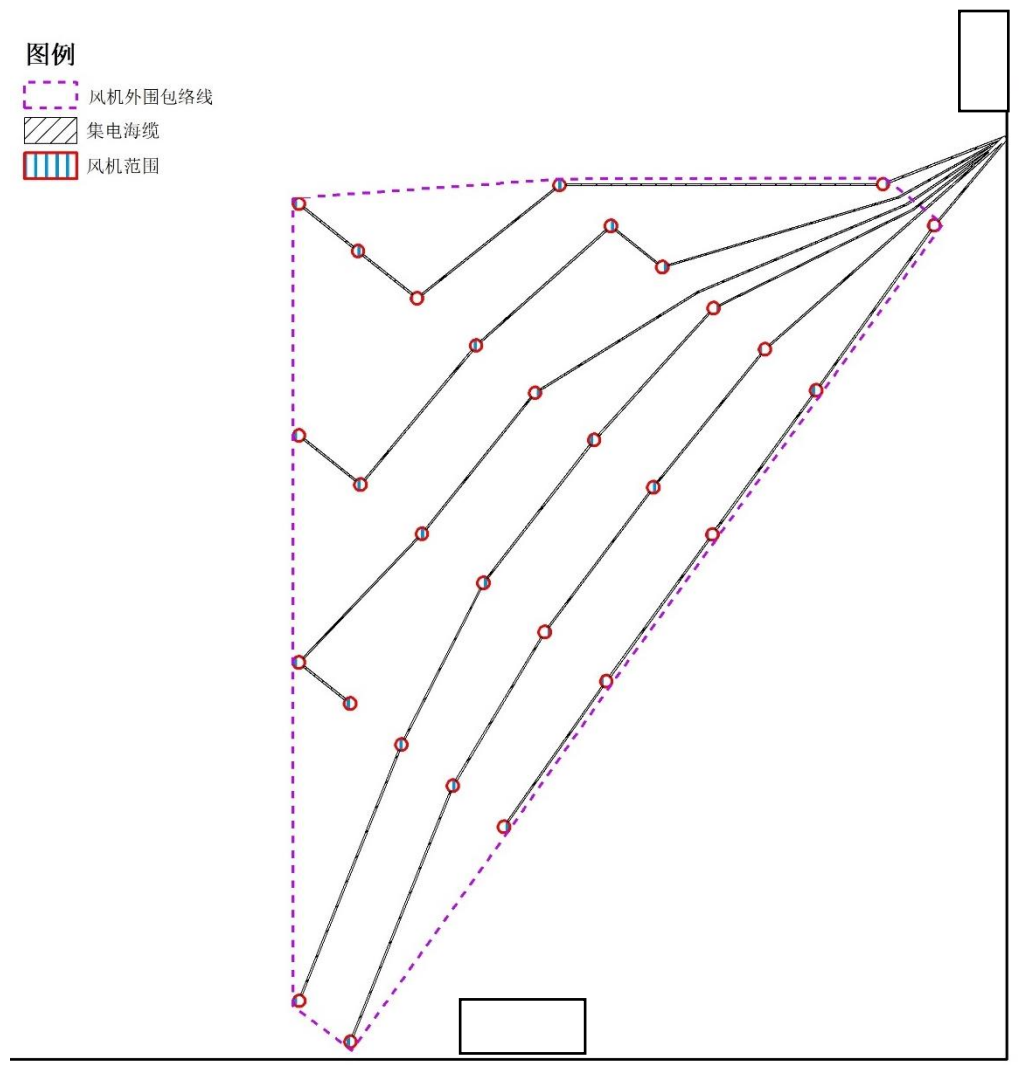
图 7.5.1-3 风机外围包络线示意图
