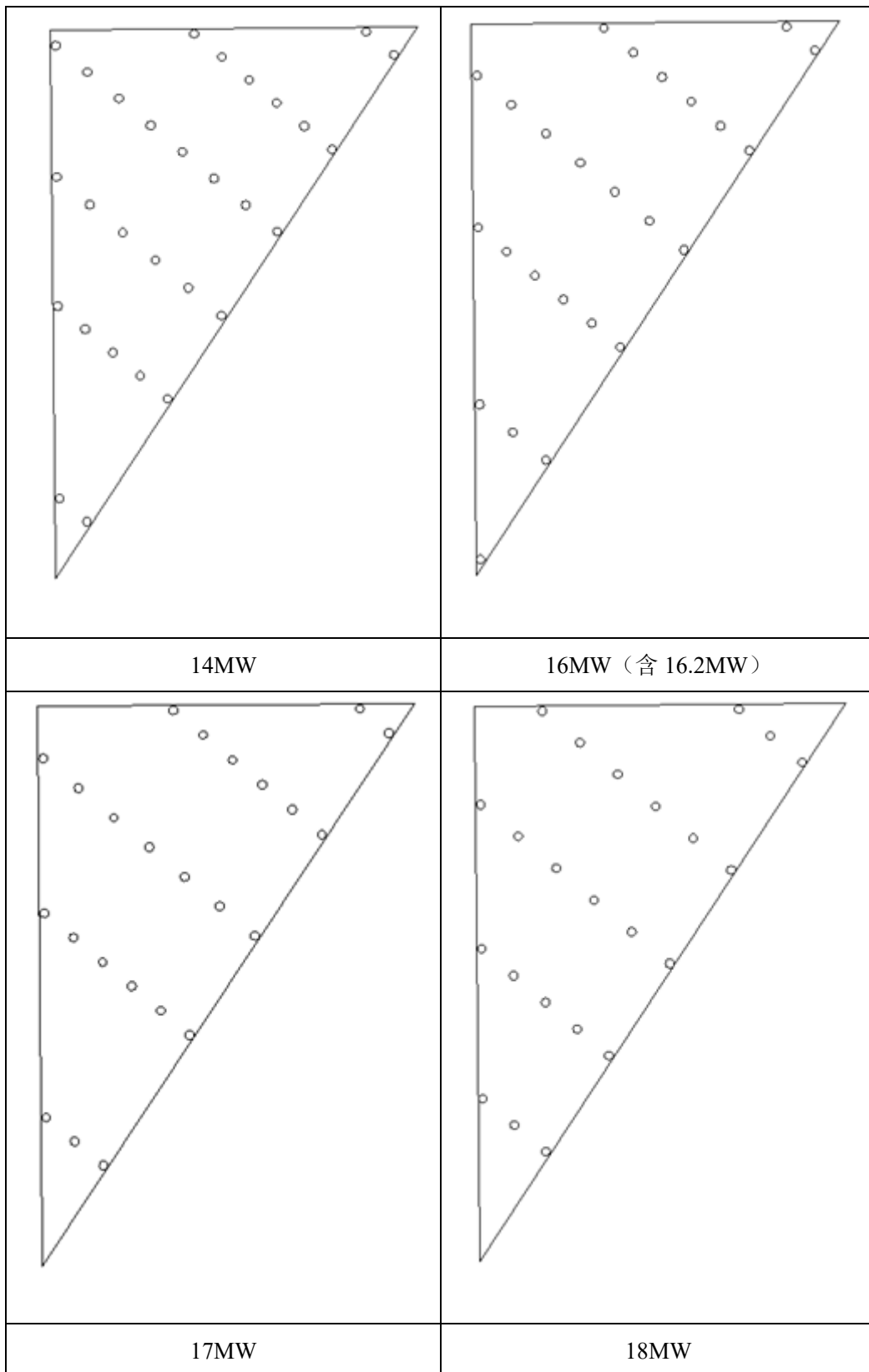
图 7.2.1-1 各容量风机机位布置示意图
