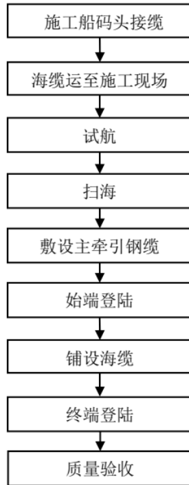
图 2.3.1-6 海缆敷设施工工艺
