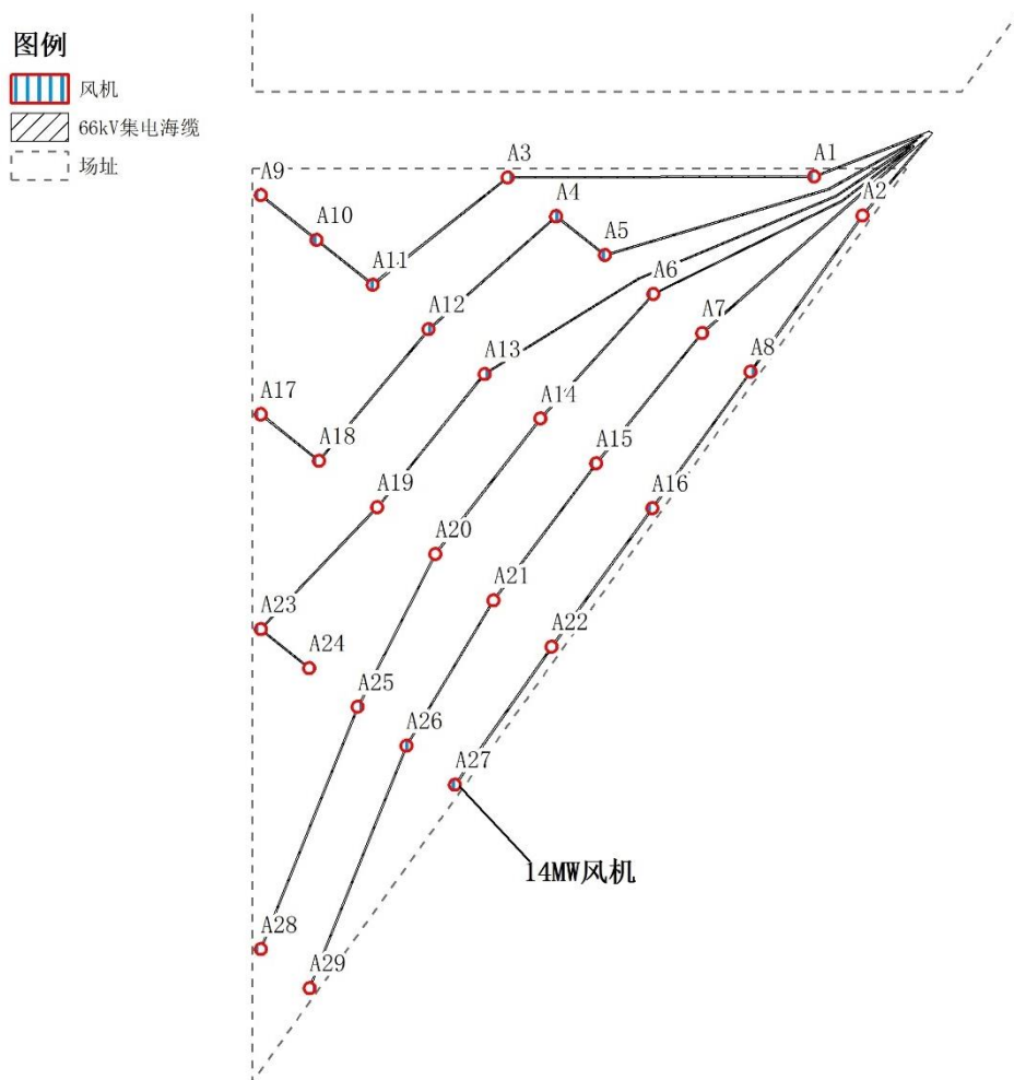
图 2.2.1-2 项目平面布置示意图
