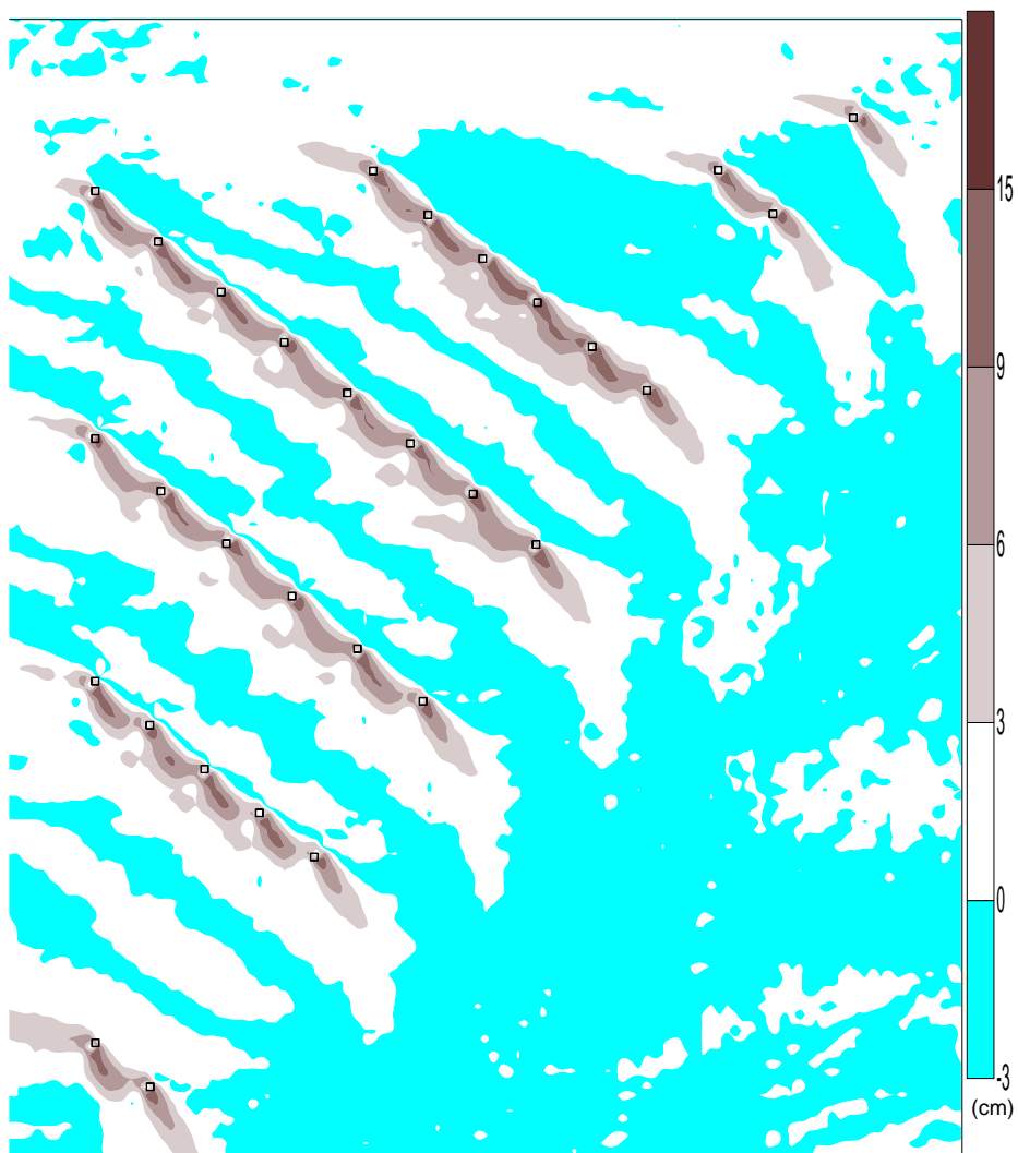
图 4.1.5-1 项目建成后冲淤平衡图
