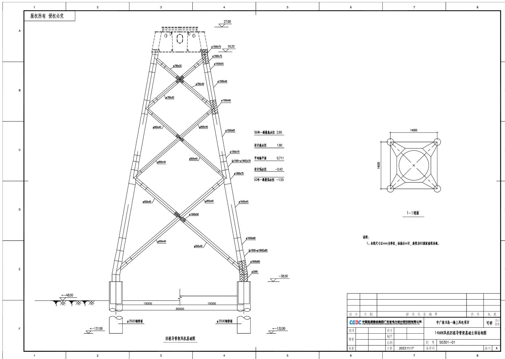
图 2.2.2-1 四桩导管架基础结构图
