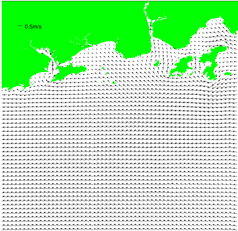
图 4.1.4-6 NE 季风环流影响下粤西大潮表层涨急流场
