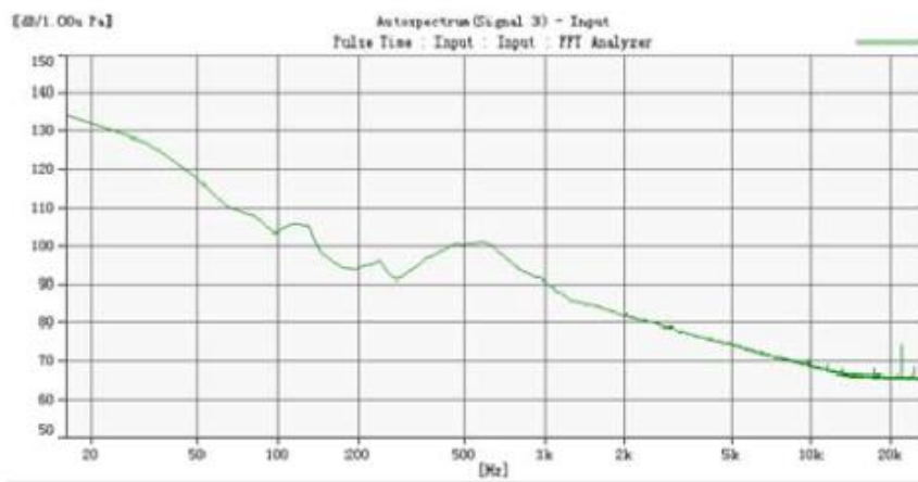
声功率谱图
