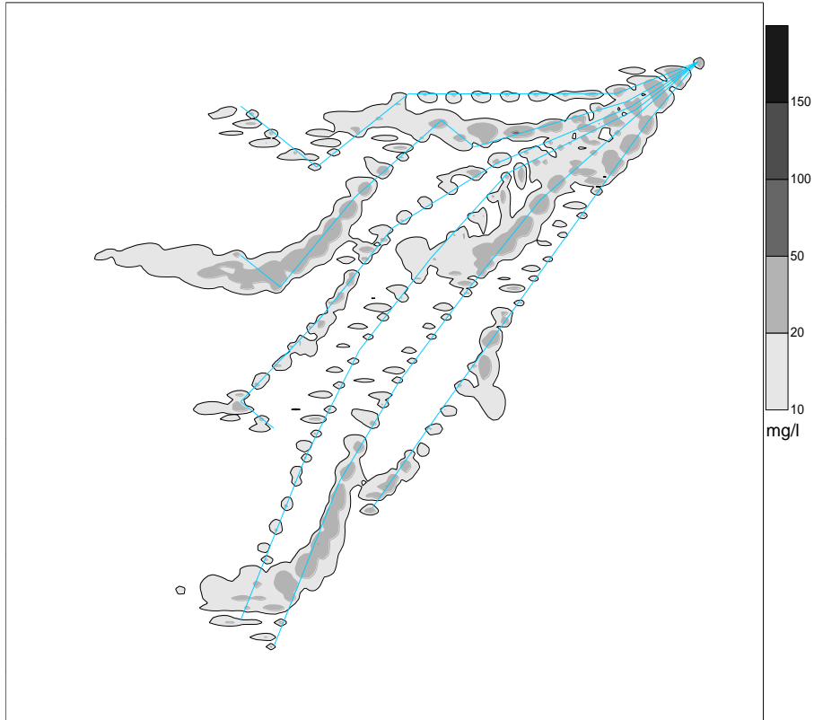
图 4.1.6-3 方案一 66kV 电缆铺缆次底层悬沙增量包络线 (大于 10mg/L 面积 18.337km 2 )
