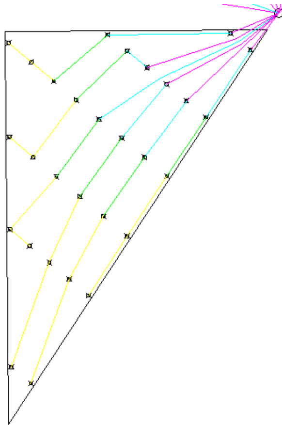
图 7.2.1-2 集电线路布置方案一
