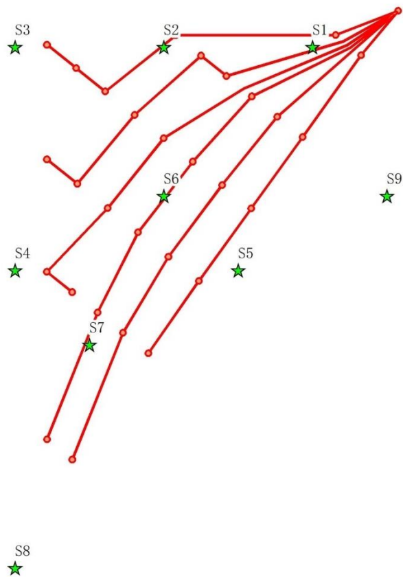
图 8.1.2-2 水下噪声监测站位图
