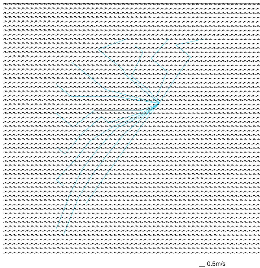
图 4.1.4-9 NE 季风大潮中层涨急流场
