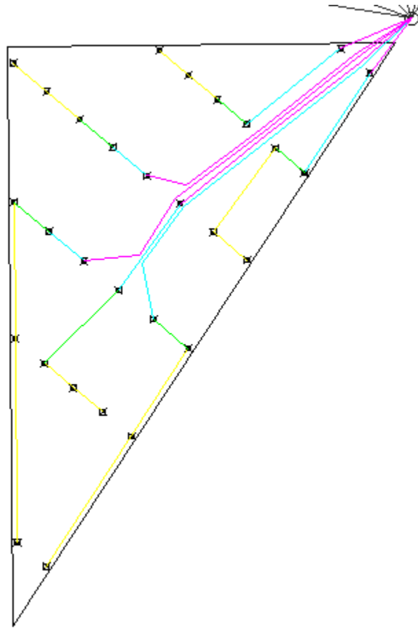
图 7.2.1-3 集电线路布置方案二
