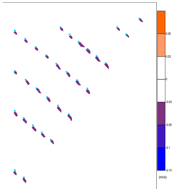
图 4.1.4-19 风电场中层落急流速变化图
