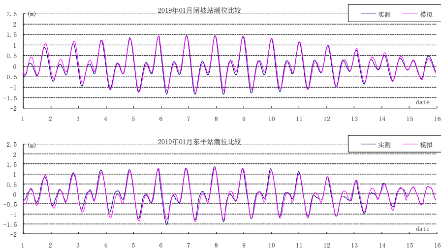
图 4.1.4-4 2019 年 1 月闸坡、东平实测与模拟潮位过程曲线
