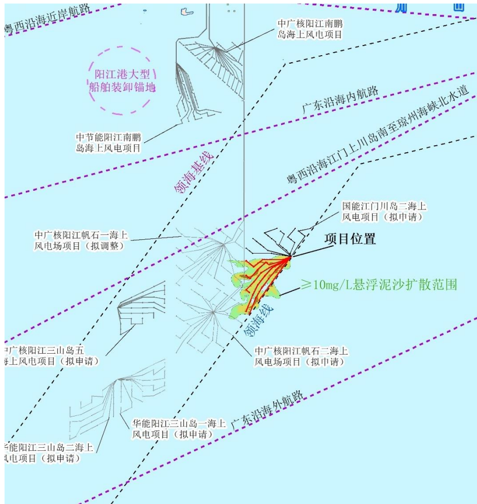
图 5.2-1 大于 10mg/L 悬沙增量包络线（底层）与周边开发利用活动叠置图
