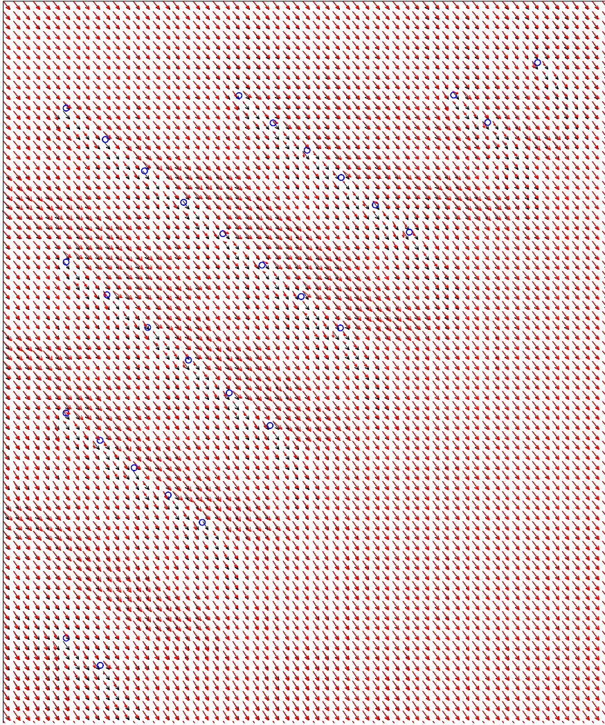
图 4.1.4-18 风电场中层落急流速对比图（黑：工程前，红：工程后）
