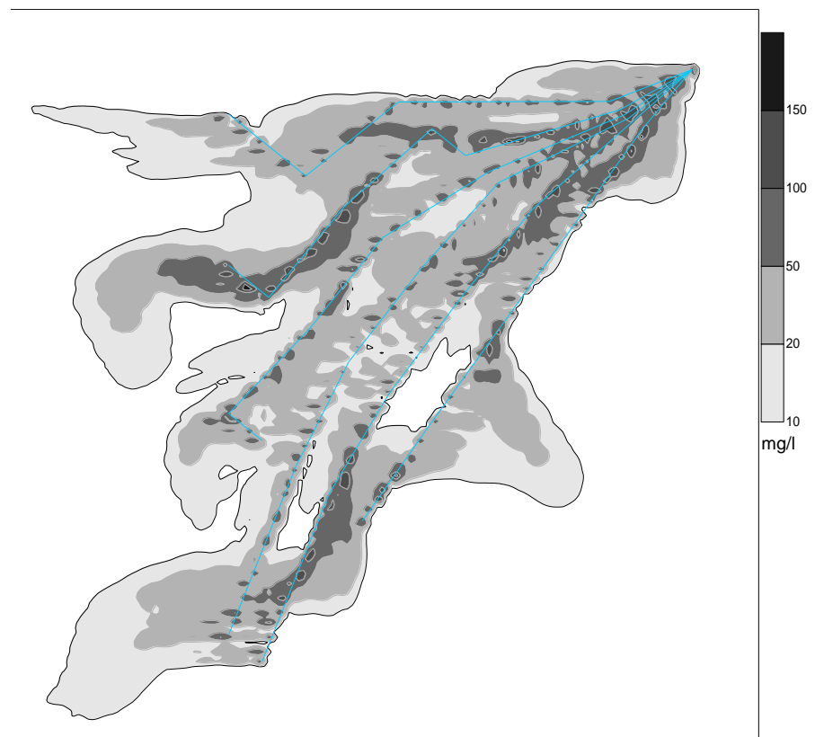
图 4.1.6-4 方案一 66kV 电缆铺缆底层悬沙增量包络线 (大于 10mg/L 面积 67.550km 2 )
