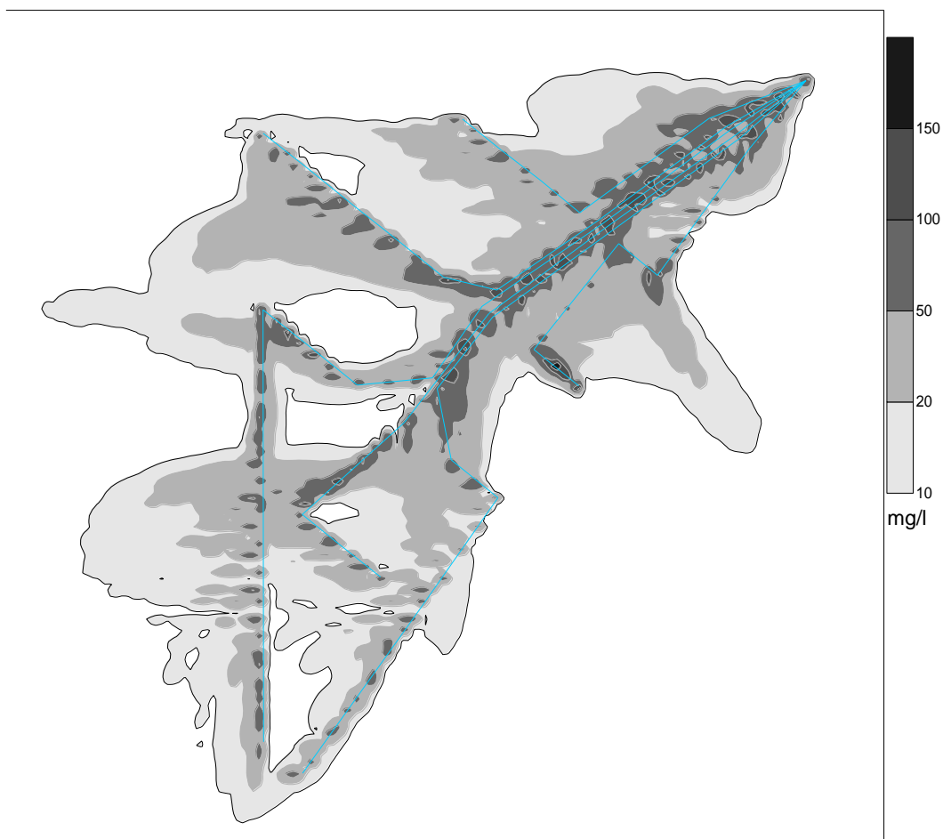
图 4.1.6-4 方案二 66KV 电缆铺缆底层悬沙增量包络线（大于 10mg/L 面积 59.725km 2 ）
