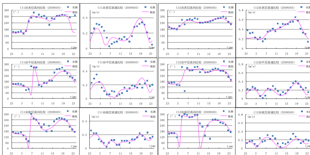
图 4.1.4-5 2019 年 1 月 5 日大潮 8 站流速流向模拟与实测比较
